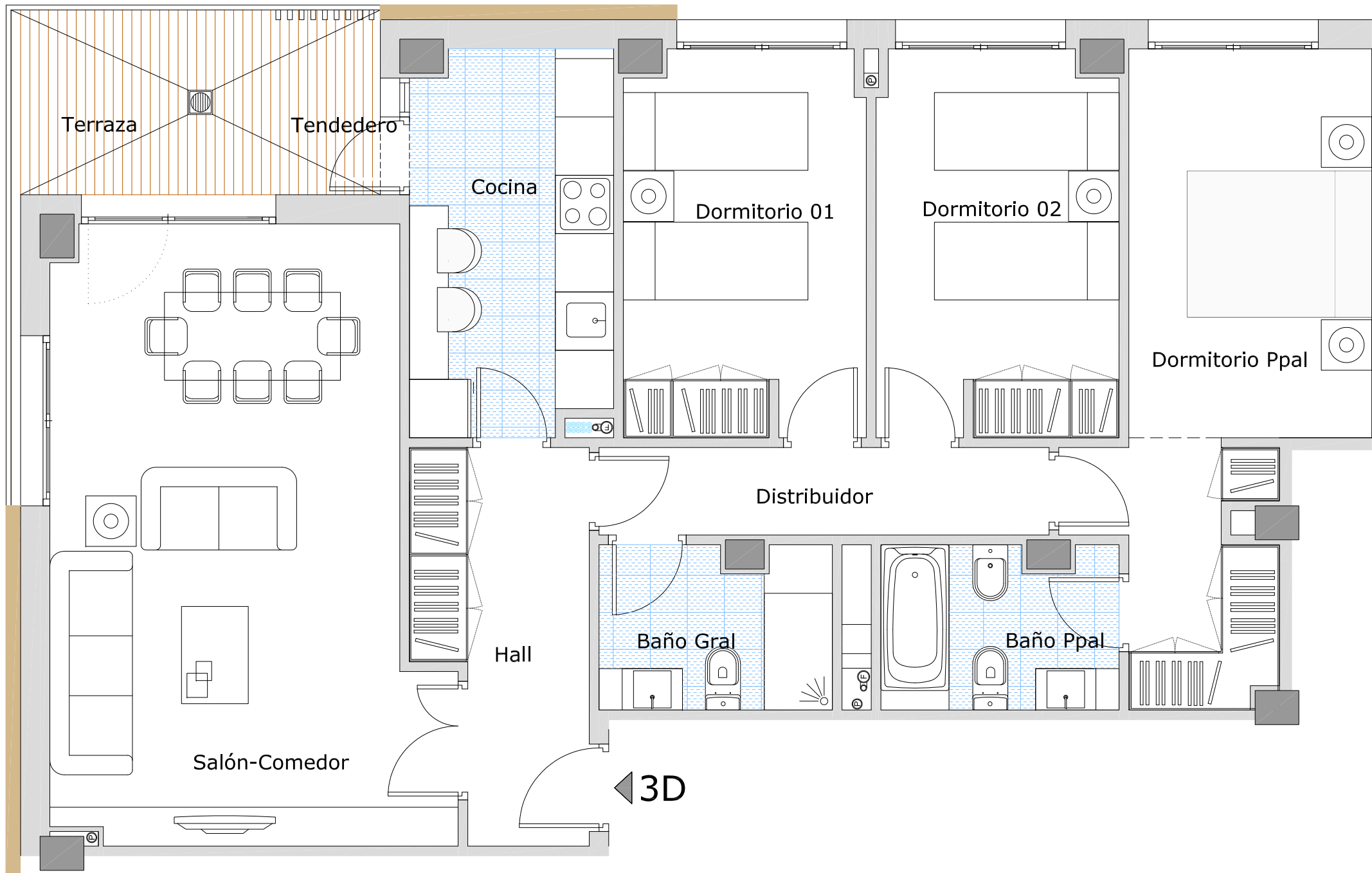
TIPO 07 PLANTAS 1 A 5
